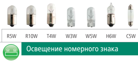
R5W R10W T4W W3W W5W H6W C5W
